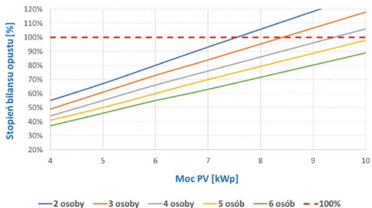
Rys. 4. Wskaźnik samowystarczalności WSW [%] w budynku o powierzchni 200 m² w standardzie NF 40 w zależności od mocy instalacji PV i liczby domowników
