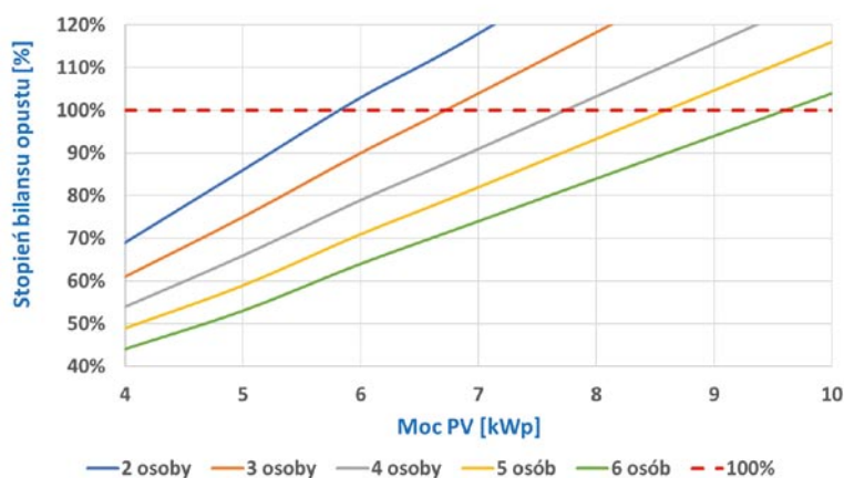
Rys. 2. Wskaźnik samowystarczalności WSW [%] w budynku o powierzchni 100 m² w standardzie NF 40 w zależności od mocy instalacji PV i liczby domowników
